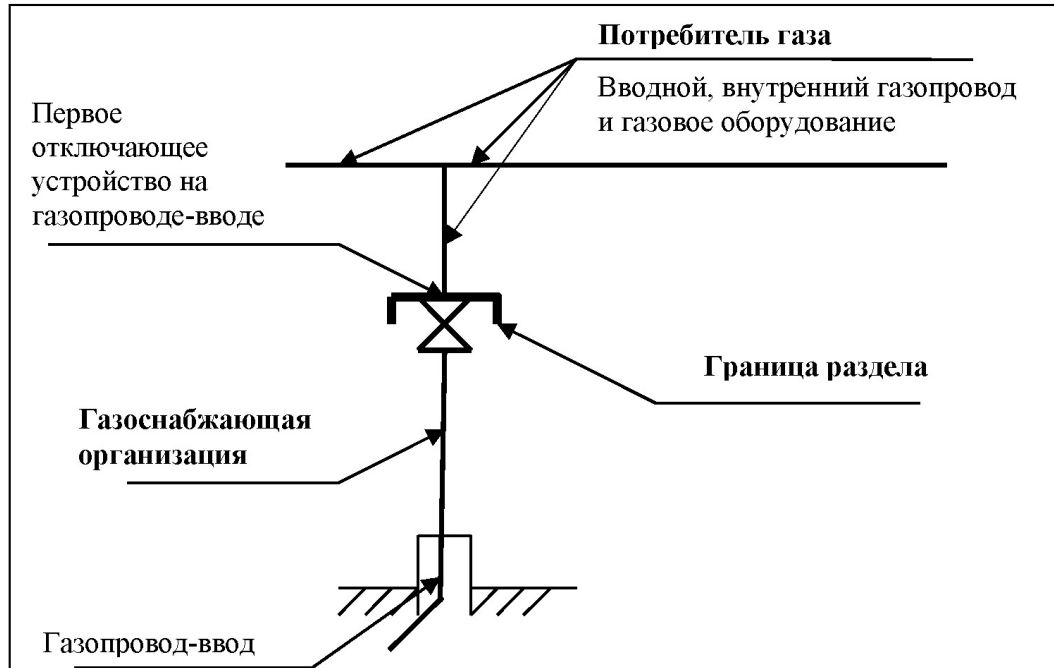
Примерная схема
