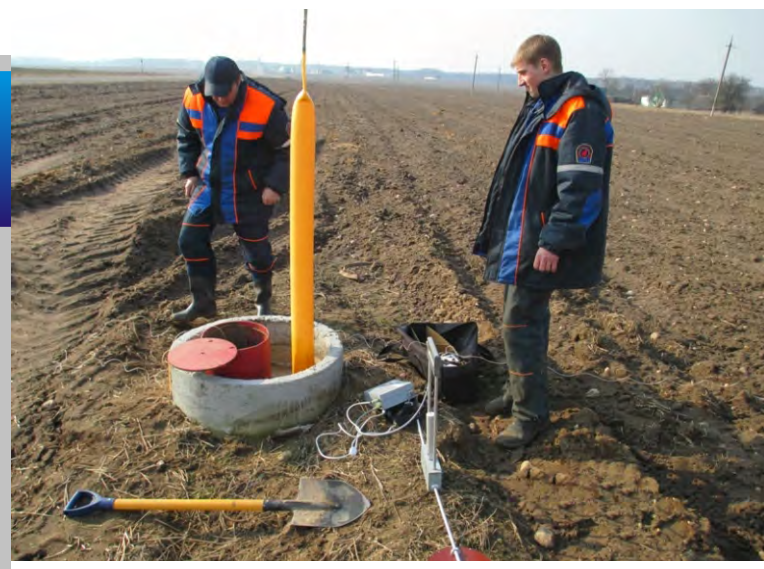
Слесарь УЗГ Ерш В.В. и слесарь СОРНГГО Кот А.А. обследуют газопровод на повреждения изоляции.
